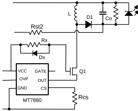
图 3、通过 VCC 驱动外部功率 MOS 管
