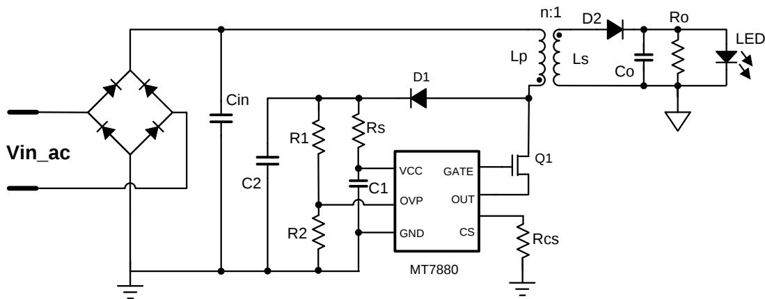
图 4、隔离反激式应用电路图
