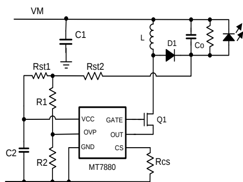
图1、OVP 设置
