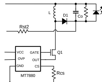
图2、内部驱动电路直接驱动
