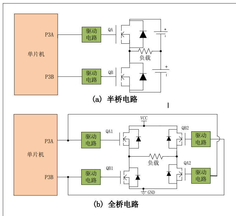
图 8.7 半桥输出模式应用举例
