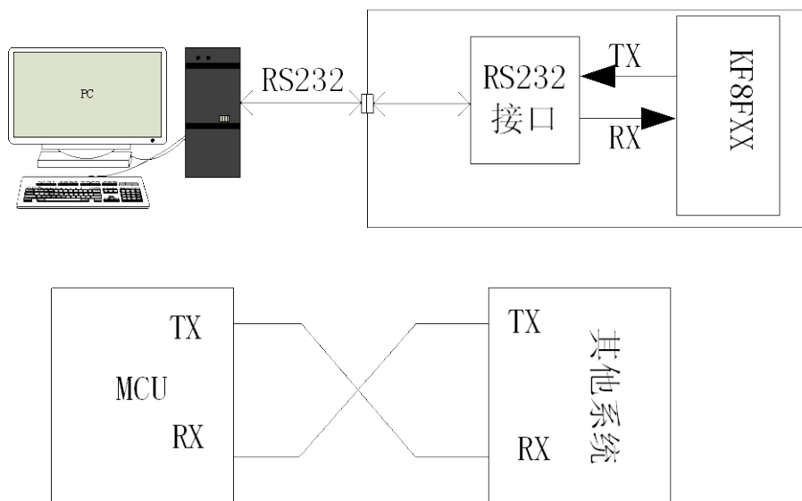
图 11.5 串口通信原理框图
