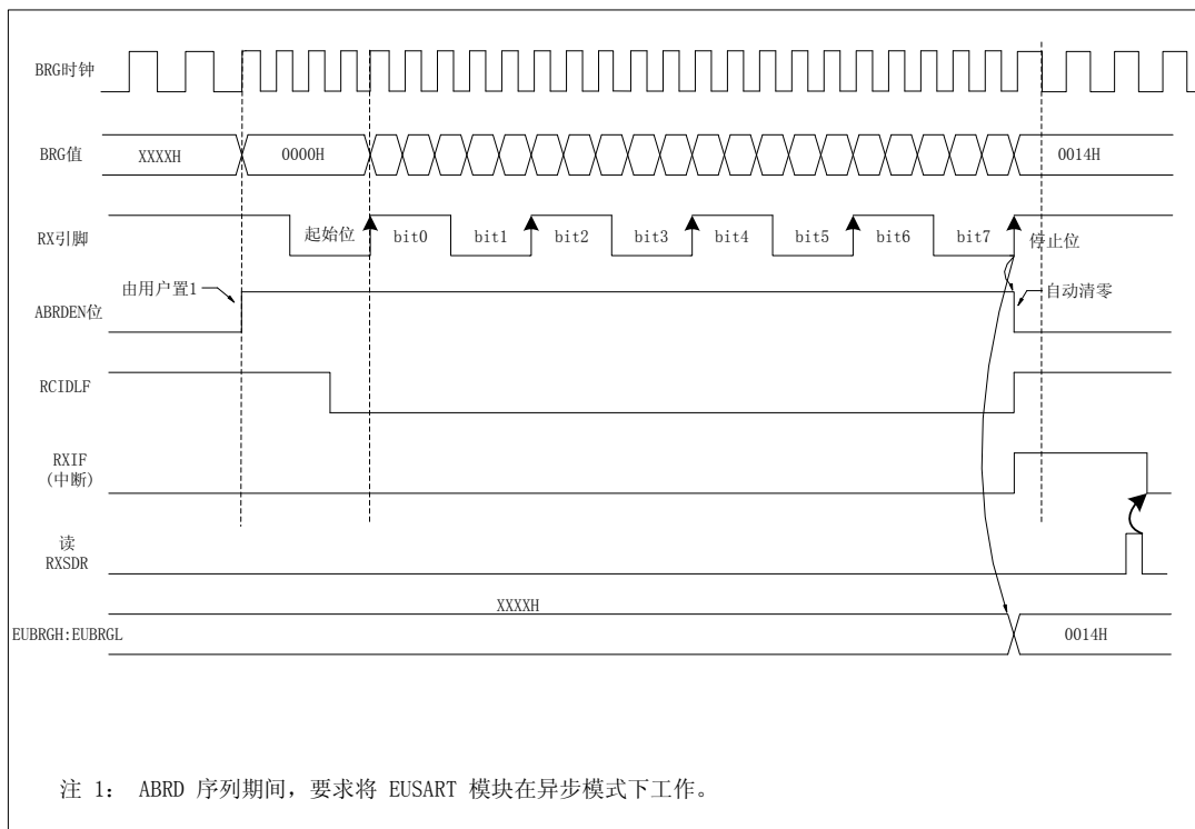
图 11.3 自动波特率检测
