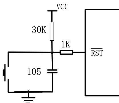
图 12.2 建议 \overline{\text{RST}} 复位电路
