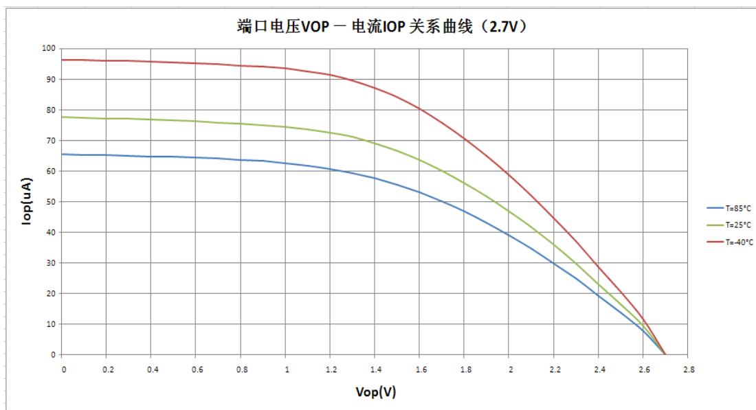
图16-13: 上拉功能打开时端口电压 V_{OP} — 电流 I_{OP} 关系曲线图 ( V_{DD} = 2.7V )
