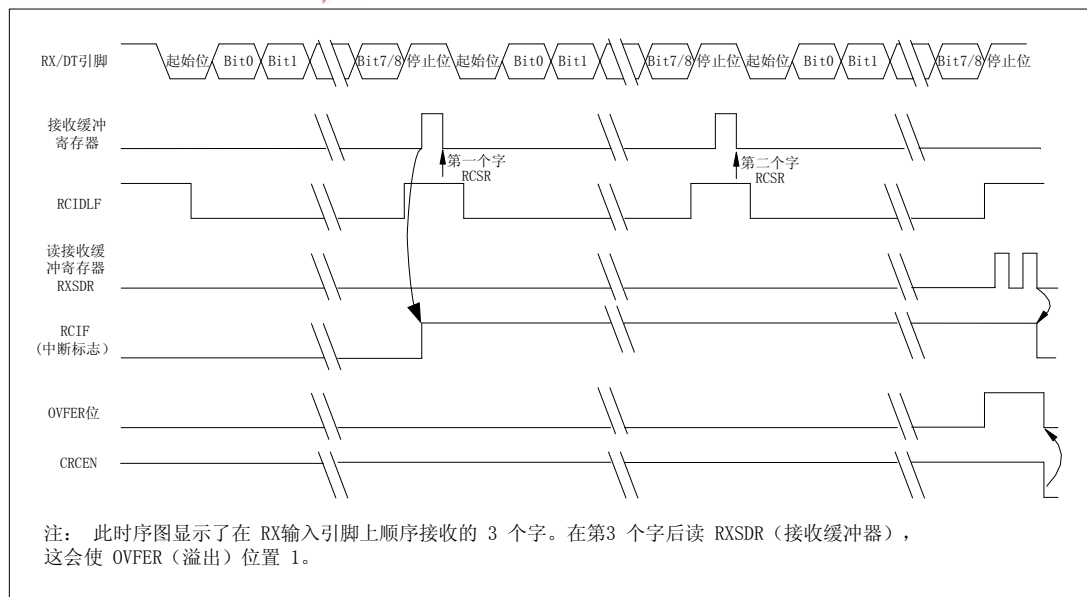
图 11.8 全双工异步接收
