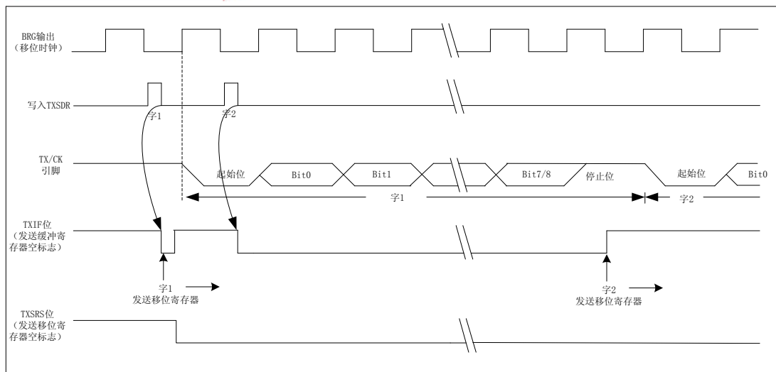
图 11.7 全双工异步发送（一字符接一字符）
