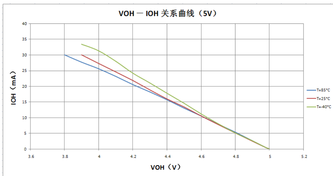
图16-8: 不同温度时 V_{OH} — I_{OH} 关系曲线图 ( V_{DD} = 5.0V )
