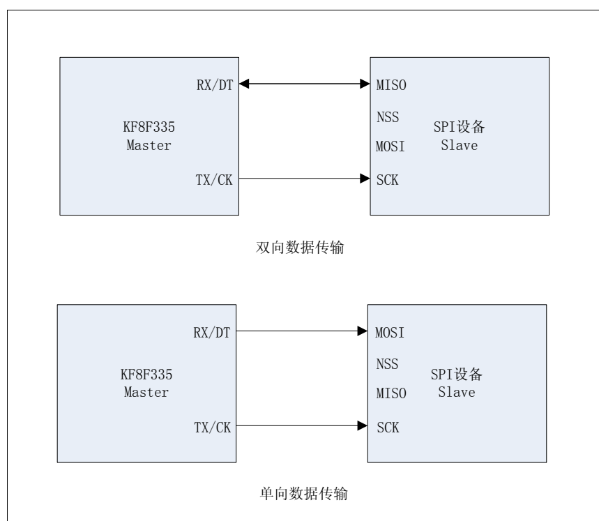
图 11.15 SPI 单线传输图
