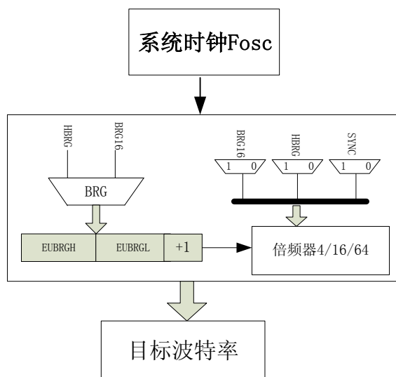
图 11.2 目标波特率产生原理框图
