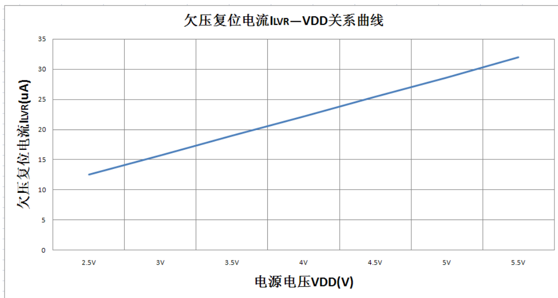
图 16-7: 欠压复位电流 I_{LVR} — V_{DD} 关系曲线图
