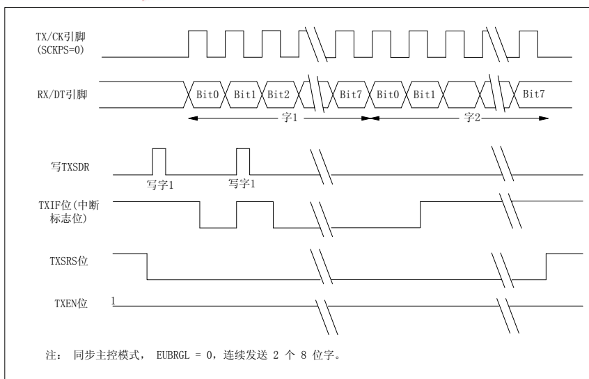
图 11.9 半双工同步发送 (SCKPS=0)
