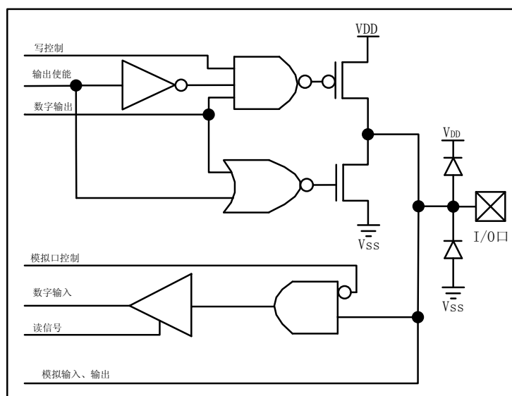
图 2.5 P2 口引脚原理功框图
