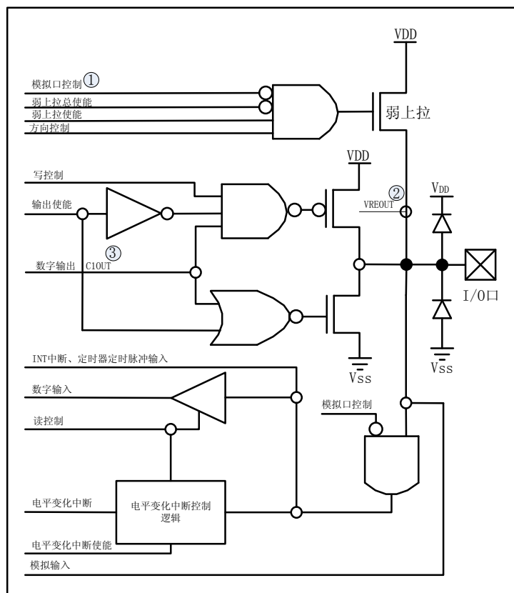
图 2.3 引脚 P0.0~P0.2、P0.4~P0.7 原理功框图
