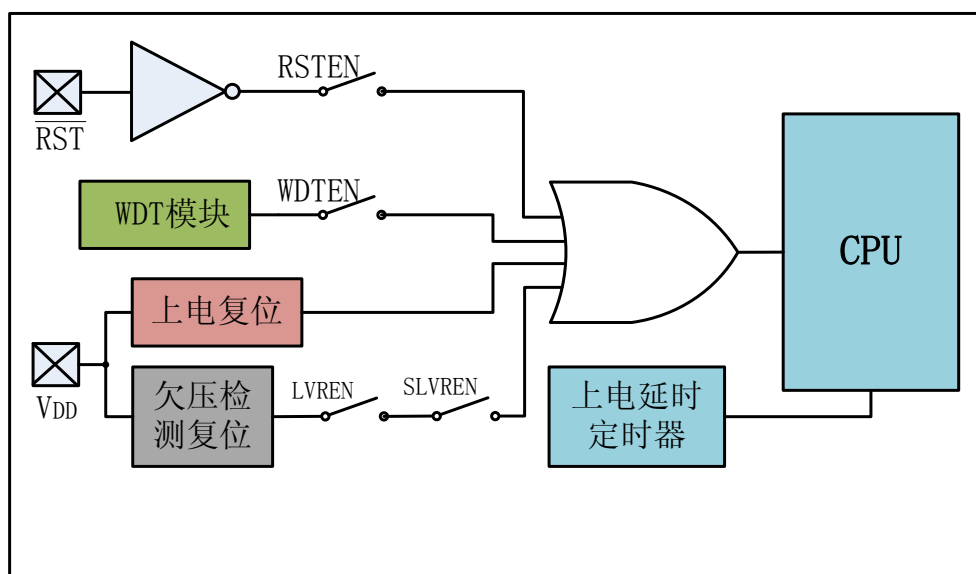
图 12.1 片内复位电路简化框图
