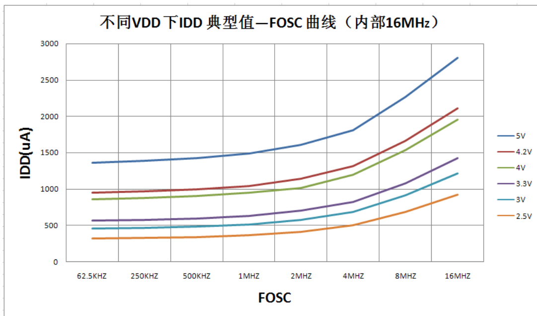
图16-1： 不同VDD 时典型IDD — FOSC 关系曲线图
