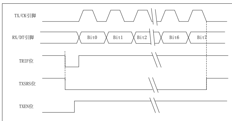
图 11.11 半双工同步发送 (通过 TXEN)
