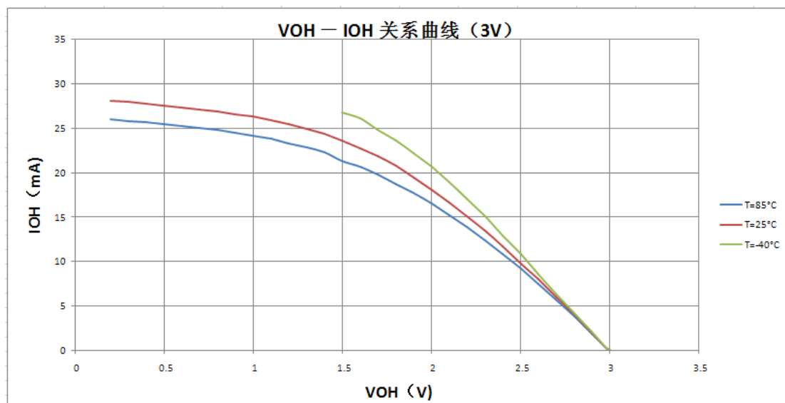
图16-9: 不同温度时 V_{OH} — I_{OH} 关系曲线图 ( V_{DD} = 3.0V )
