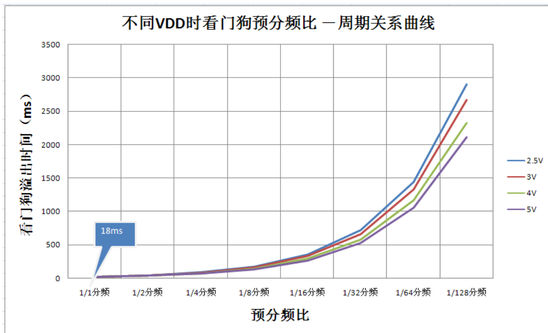
图16-4： 不同 V_{DD} 时看门狗预分频比 — 周期关系曲线图
