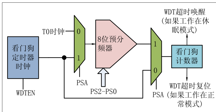
图 14.1 看门狗定时器框图
