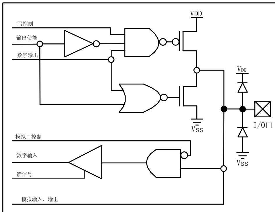
图 2.6 P4 口引脚原理功框图
