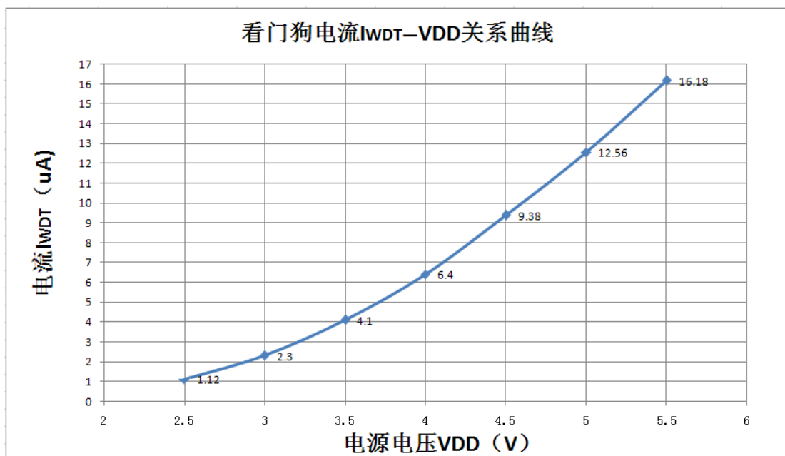
图16-5: 看门狗电流 — VDD关系曲线图
