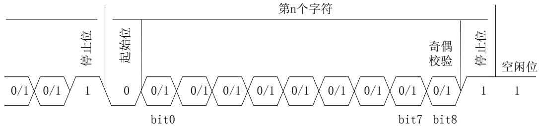
图 11.4 全双工异步通信数据结构图
