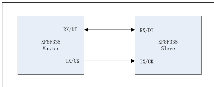
图 11.14 SPI 单线传输图
