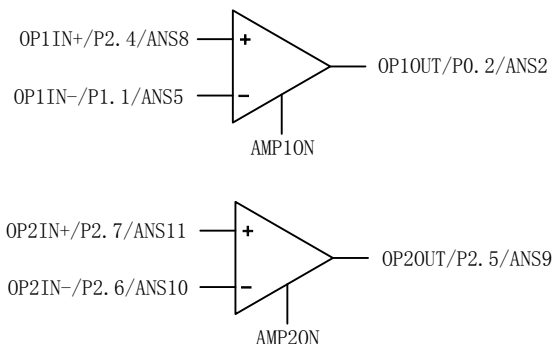
图 9.1 运放内部框图
