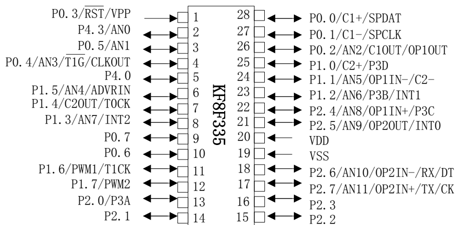
图 2.1 KF8F335 引脚功能图
