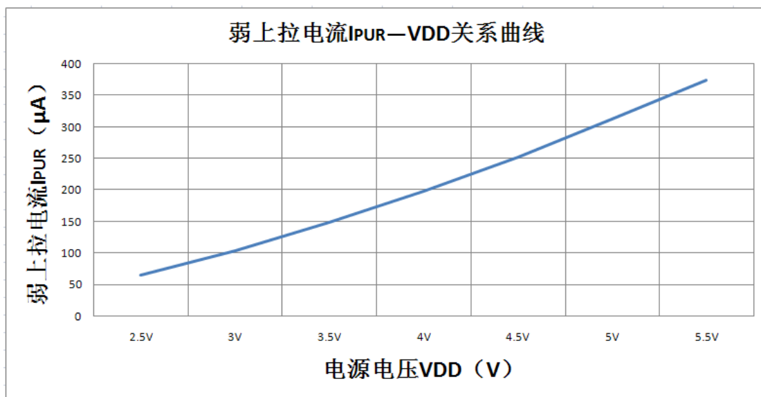
图16-3： 弱上拉电流 I_{PUR} — V_{DD} 关系曲线图
