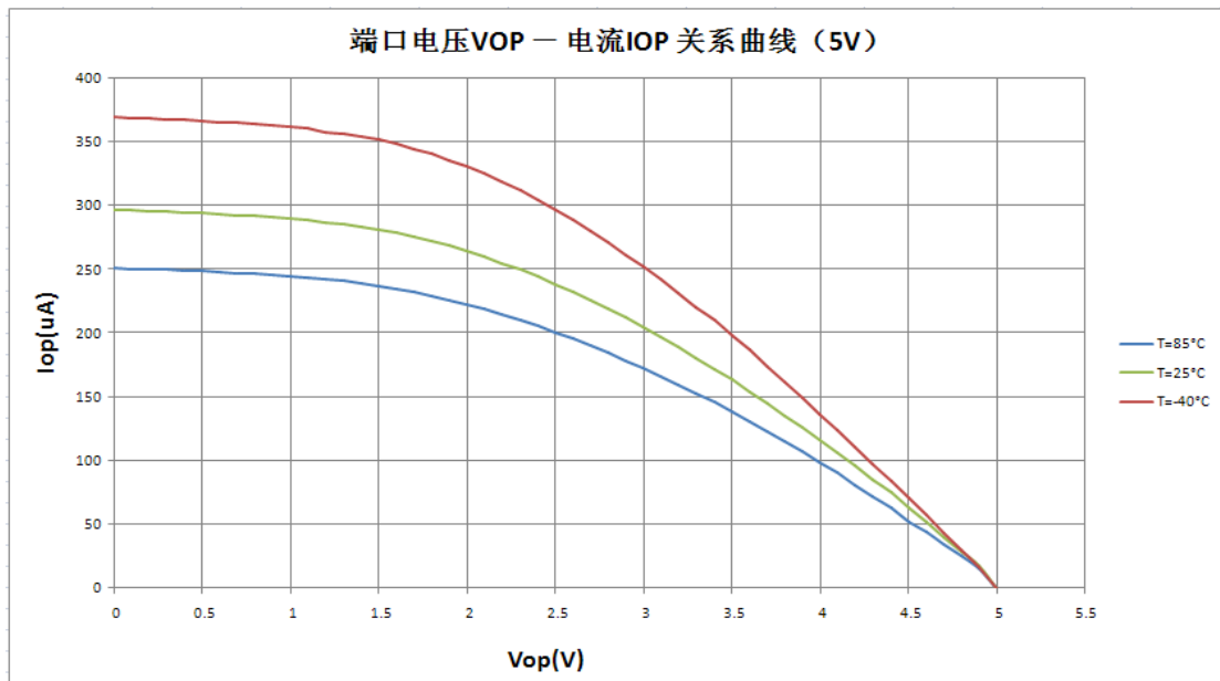
图16-12: 上拉功能打开时端口电压 V_{OP} — 电流 I_{OP} 关系曲线图 ( V_{DD} = 5.0V )
