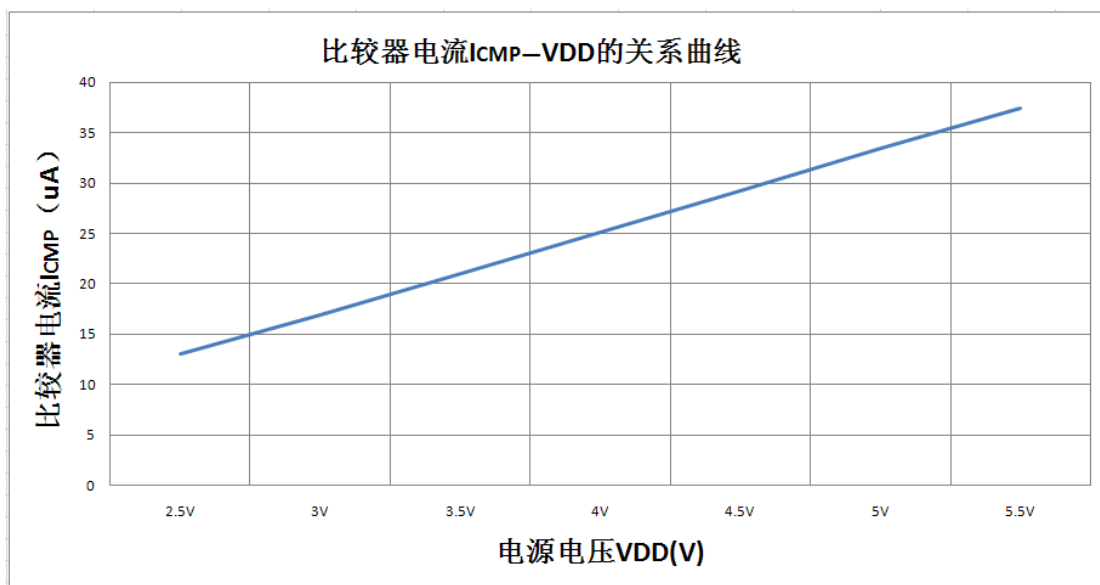
图16-6: 比较器电流 — VDD关系曲线图（使能一路比较器）
