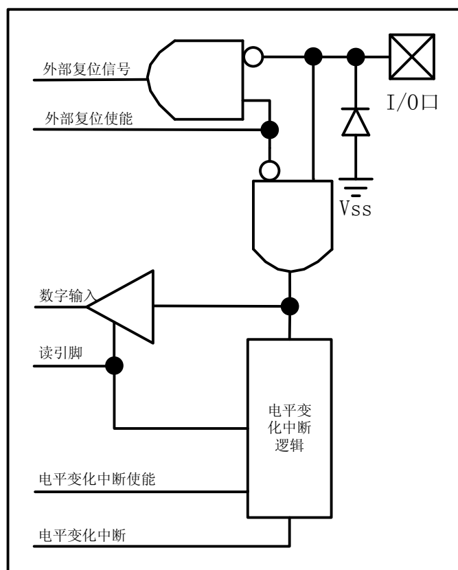
图 2.2 引脚 P0.3 内部原理功框图
