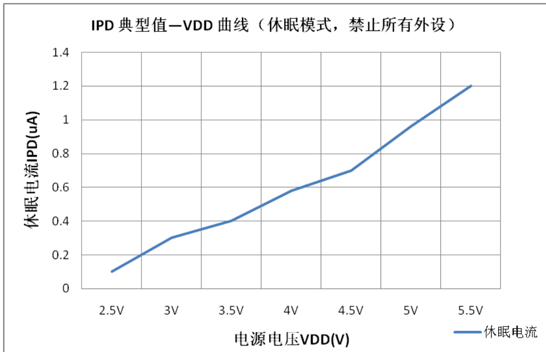
图16-2： 不同VDD 时典型IPD — VDD 关系曲线图
