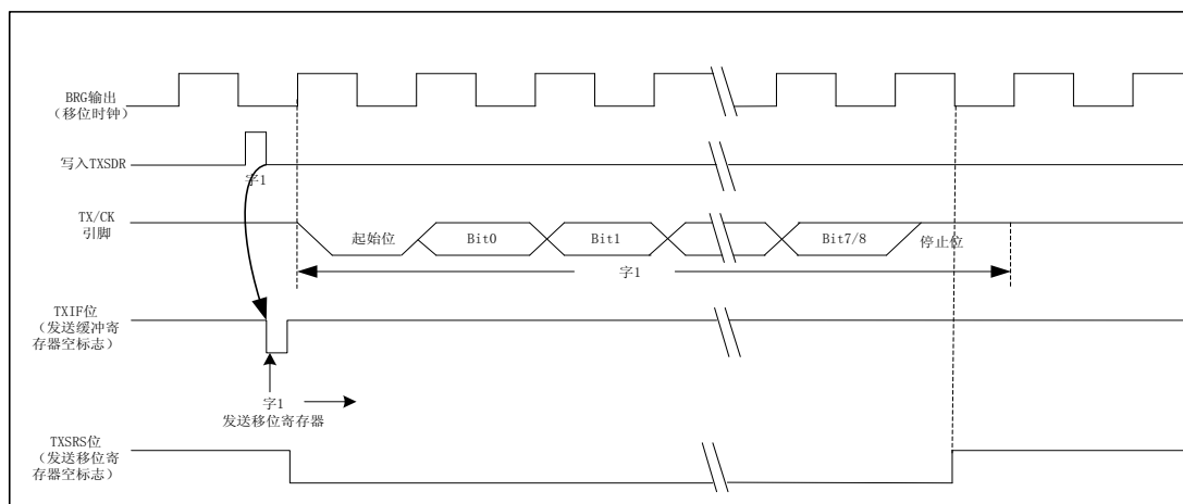
图 11.6 全双工异步发送（两字符间有空闲位）
