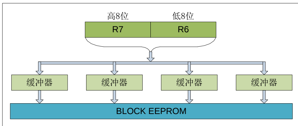
图 3.6 写操作
