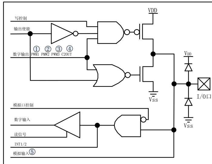
图 2.4 P1 口引脚原理框图
