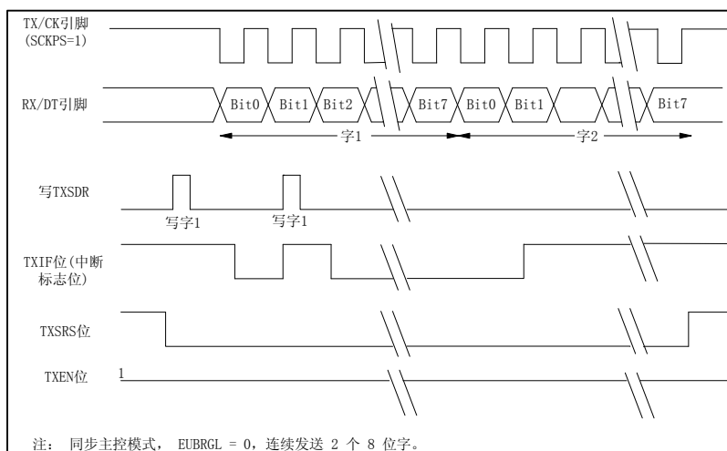
图 11.10 半双工同步发送(SCKPS=1)
