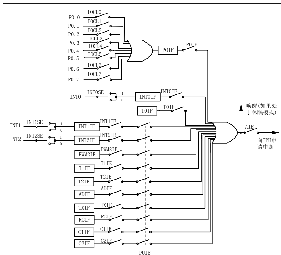
图 5.1 中断逻辑
