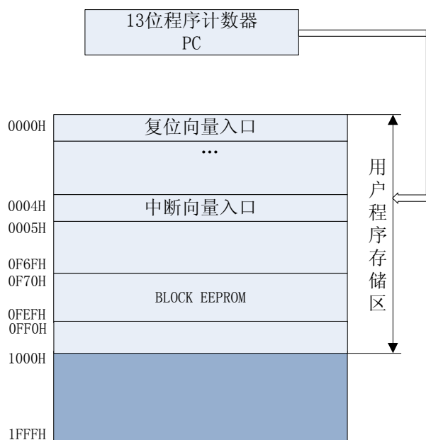
图 3.3 KF8F335 程序存储器映射
